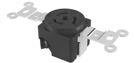
15A 250V~ Model:SRL615R
