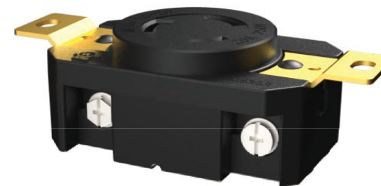
20A 250V~ Model:SRL530R
